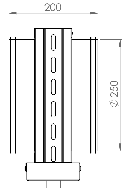
Vid Ø250 kanalsystem
